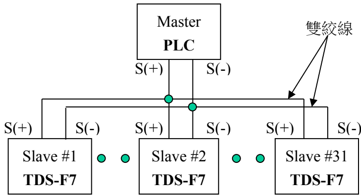
圖1：RS-485接線
