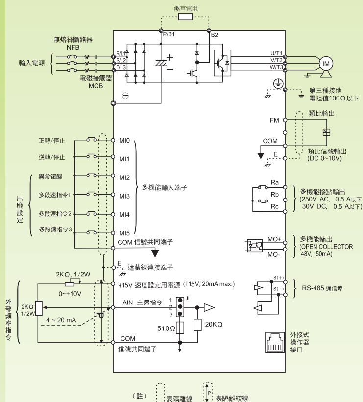
TDS-F8 變頻器標準配線圖(◎表示主回路端子,○表示控制回路端子)。
